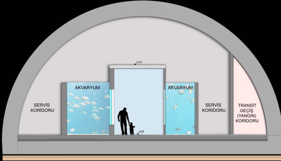
C-C KESİTİ
